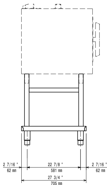
Oldalnézet
